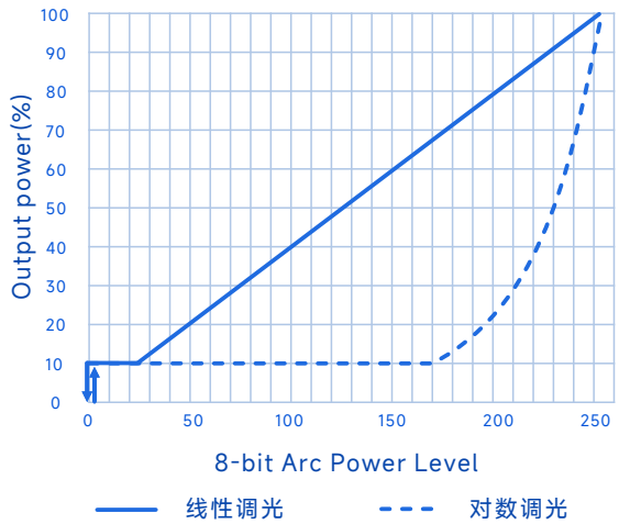
DALI调光曲线
