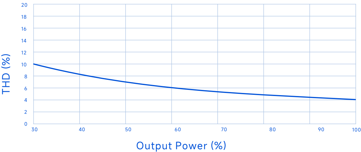
总谐波失真Vs.输出功率(Vin=230Vac)
