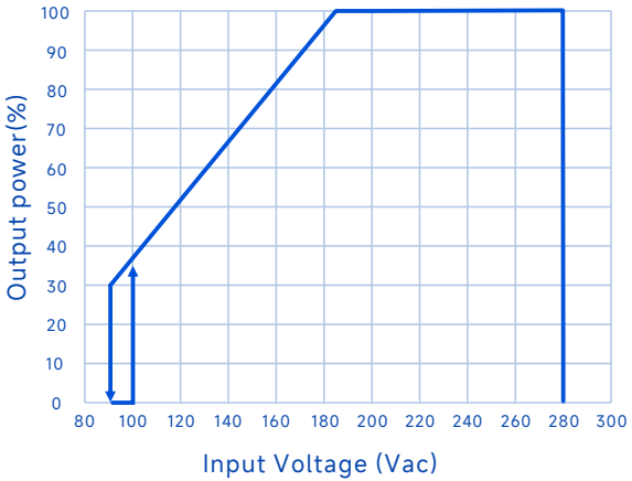
AC调光曲线
