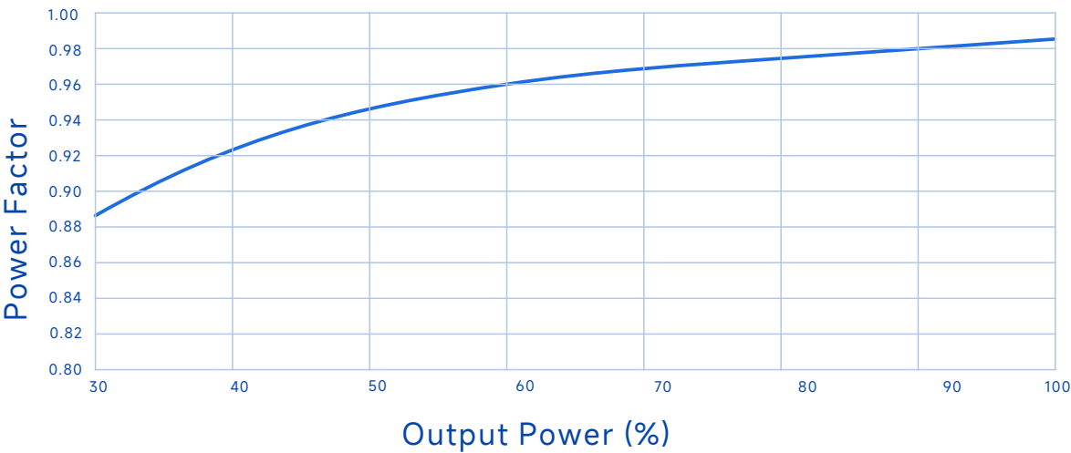
功率因数Vs.输出功率(Vin=230Vac)
